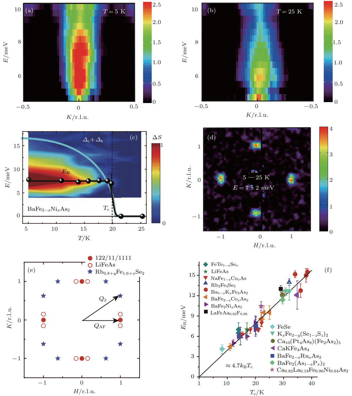
图7 (a)和(b)最佳掺杂处 \text{BaFe}_{1.904}\text{Ni}_{0.096}\text{As}_2 5 K (低于 T_c ) 和 25 K (高于 T_c ) 的低能激发; (c) 自旋共振能和超导能隙总和随温度的变化 [71] ; (d) 共振能 7 meV 附近的磁激发; (e) 五类铁基超导体自旋共振峰在动量空间的位置 [93] ; (f) 铁基超导体中共振能 E_R 与温度的关系
