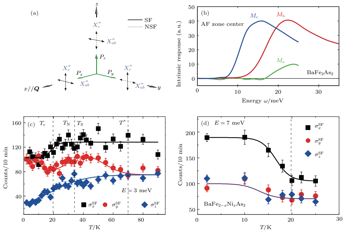
图8 (a) 中子极化方向的定义以及每个通道的磁响应 [109] ; (b) 磁布里渊区中心 M_a , M_b , M_c 的能量依赖关系 [117] ; (c), (d) Q = (0.5, 0.5, 3) 处 3 meV 和 7 meV 中子翻转散射截面 \sigma_{x,y,z}^{\text{SF}} 随温度的依赖关系
