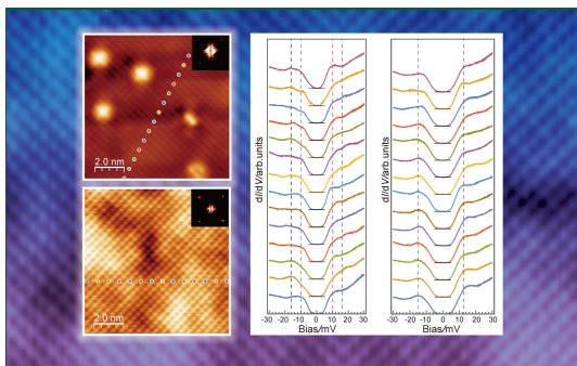
单层FeSe薄膜/氧化物界面高温超导 [丁翠, 刘充, 张庆华, 龚冠铭, 汪恒, 刘效治, 孟繁琦, 杨好好, 武睿, 宋灿立, 李渭, 何珂, 马旭村, 谷林, 王立莉, 薛其坤 2018 物理学报 67 207415]
